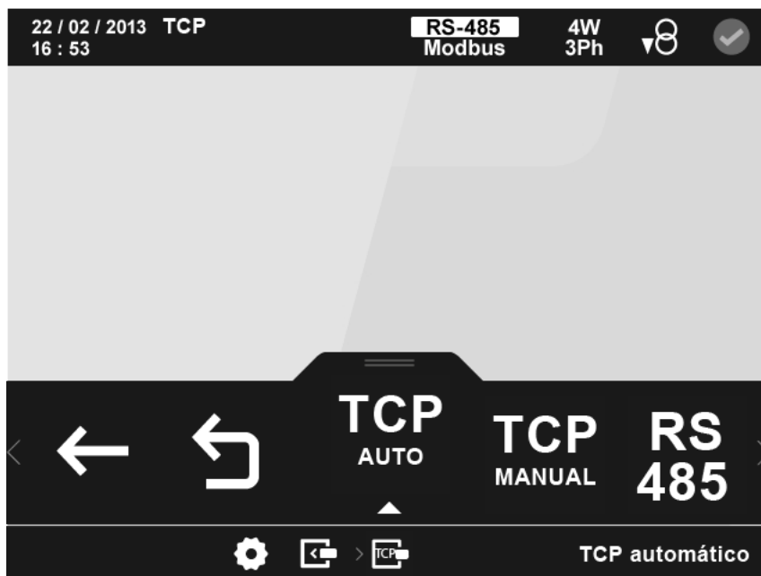
Figura 183: Pantalla principal de configuración del módulo Modbus TCP.
