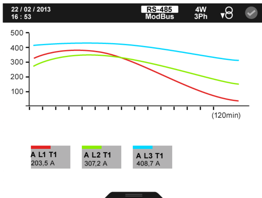
Figura 61: Parámetros de demanda, visualización gráfica (visualizar 3 parámetros).
