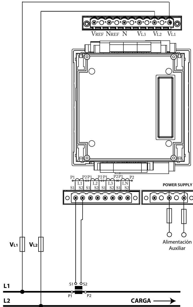
Figura 9: Medida monofásica de fase a fase de 2 hilos (Secundario del transformador: /1A, /5A o MC1 (/0.250)).
