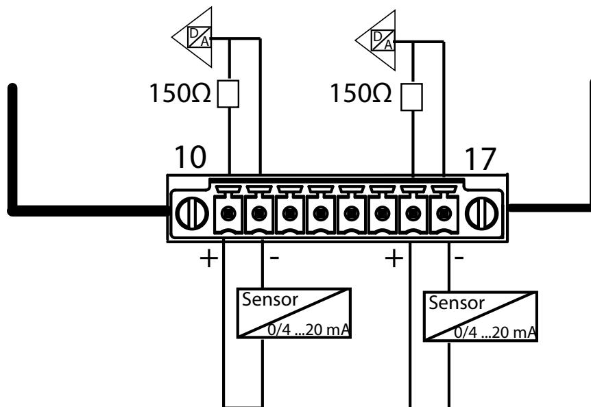
Figura 170: Esquema de conexión, entradas analógicas.
