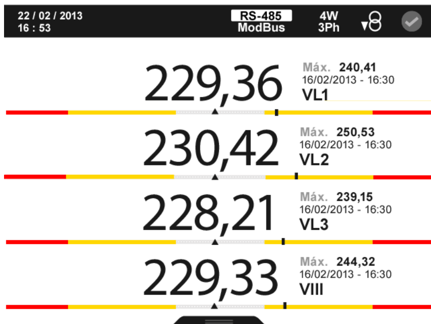
Figura 67: Parámetros instantáneos (visualizar 4 parámetros).
