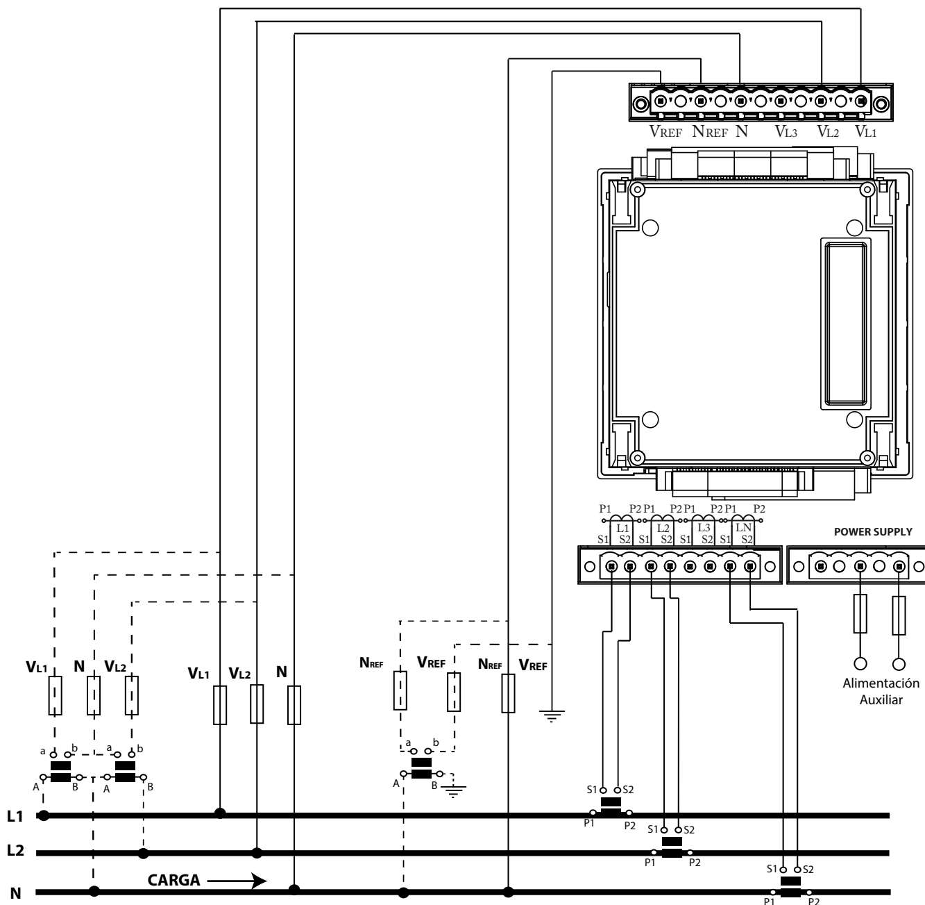
Figura 8: Medida bifásica con conexión a 3 hilos (Secundario del transformador: /1A, /5A o MC1 (/0.250)).
