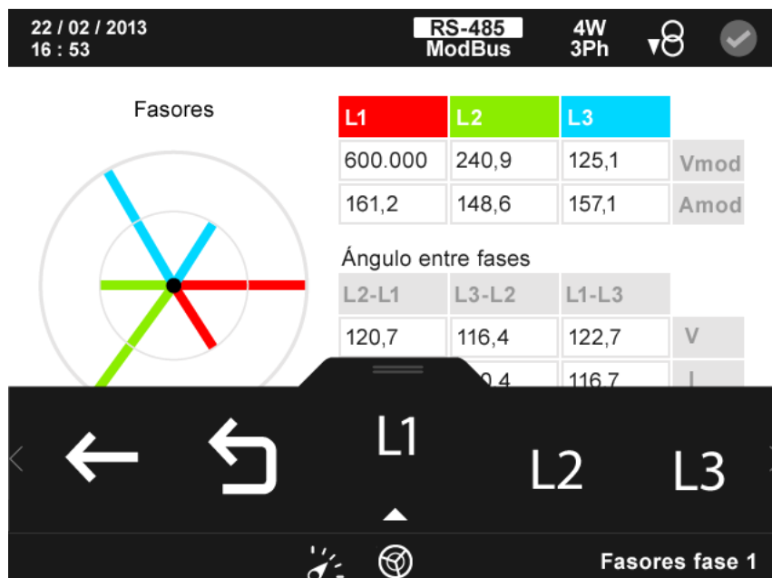
Figura 80: Pantalla de visualización de fasores.
