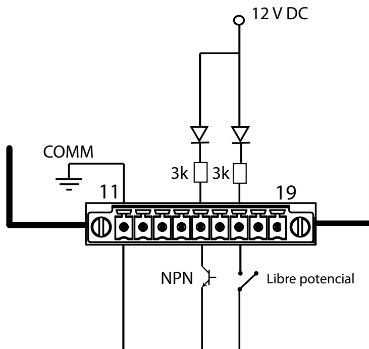
Figura 153: Esquema de conexionado, entradas digitales.
