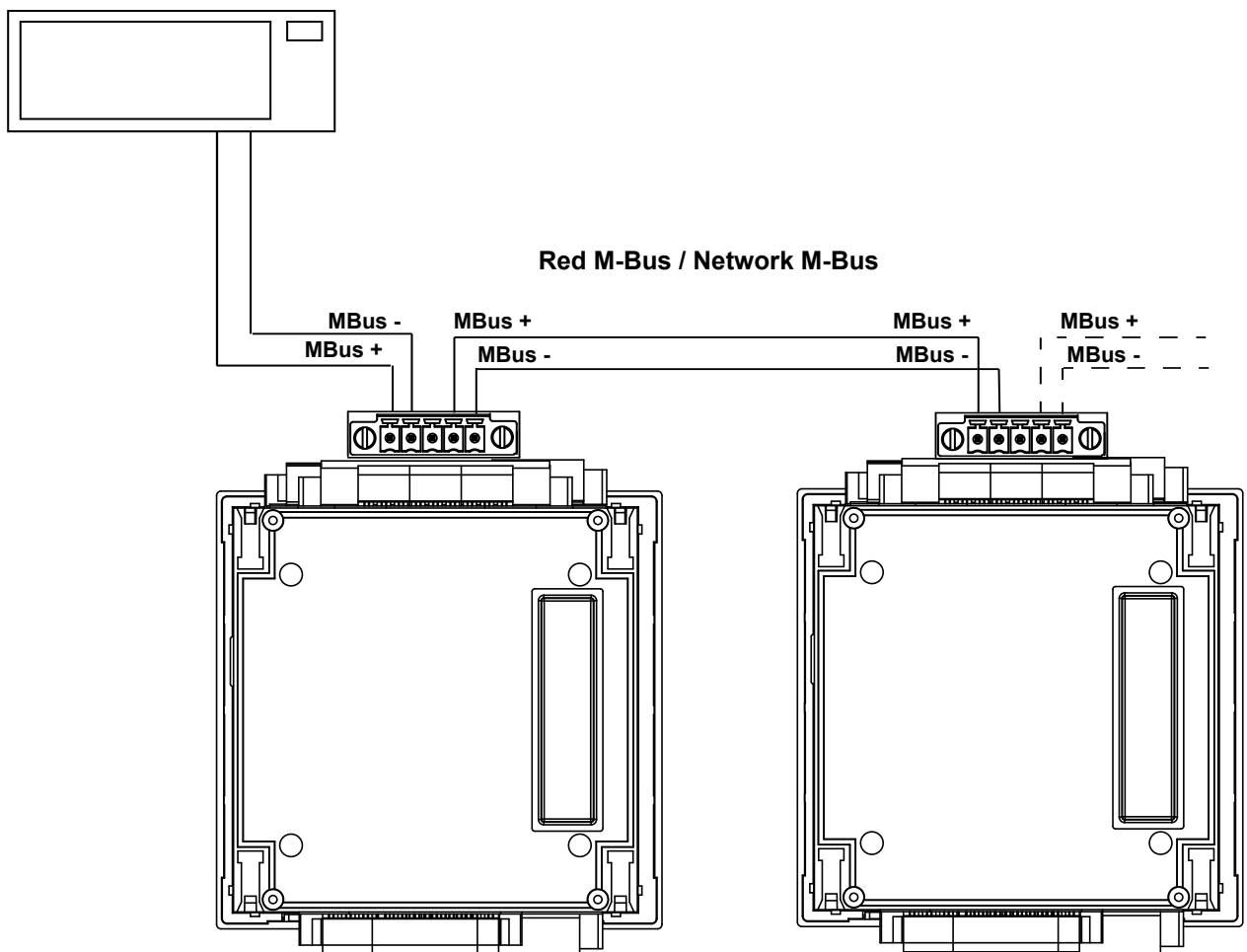
Figura 200: Esquema de conexión, MBus.
