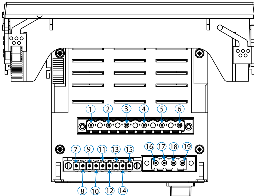
Figura 1:Bornes CVM-Bx, cara superior.
