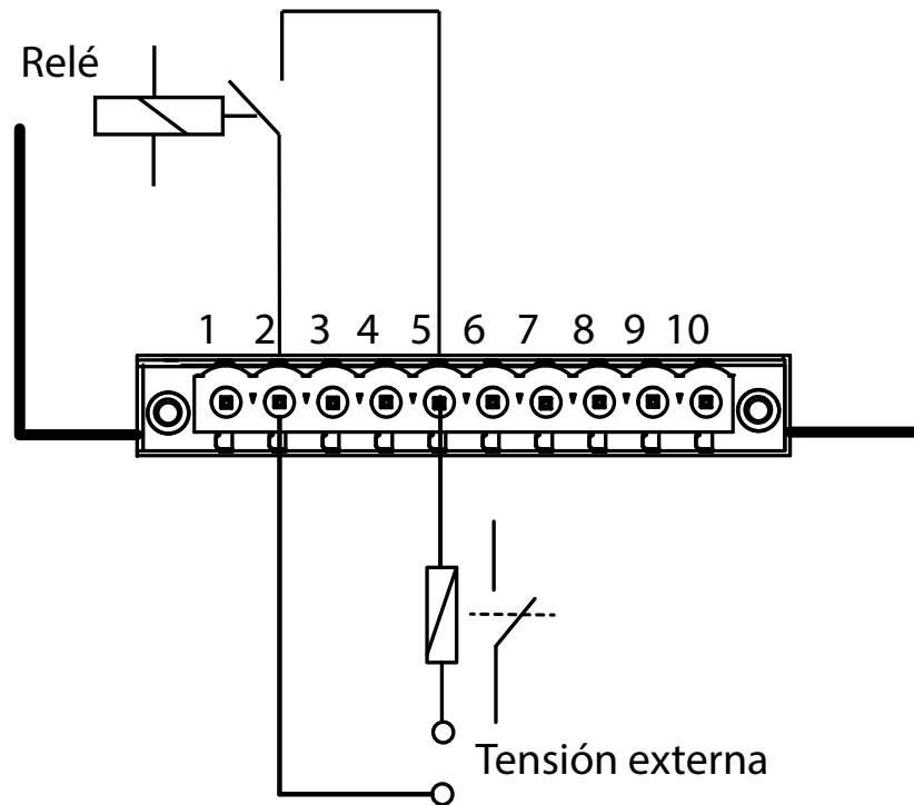
Figura 152: Esquema de conexionado, salida digitales de relé.
