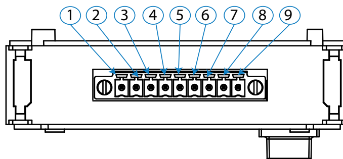
Figura 167: Bornes Entradas/Salidas analógicas, cara superior.
