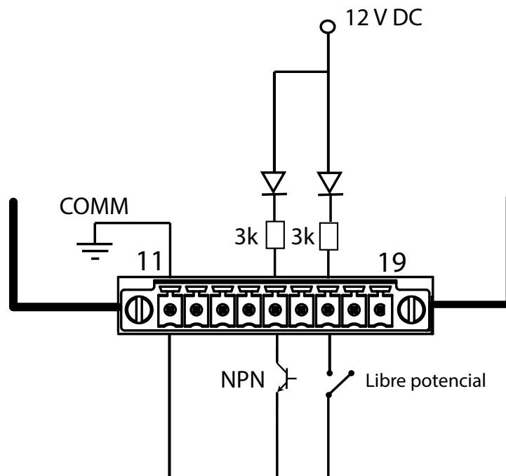
Figura 162: Esquema de conexionado, entradas digitales.
