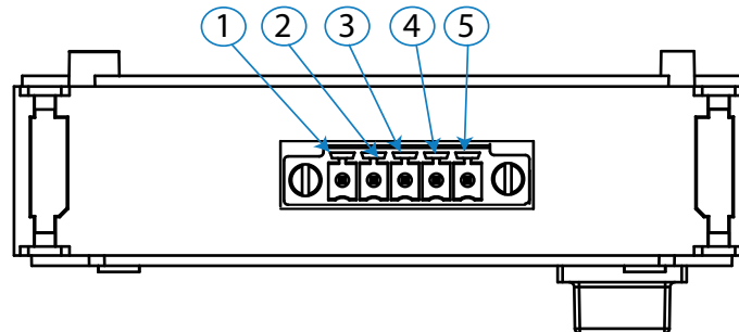
Figura 199: Bornes Módulo de comunicaciones MBus.
