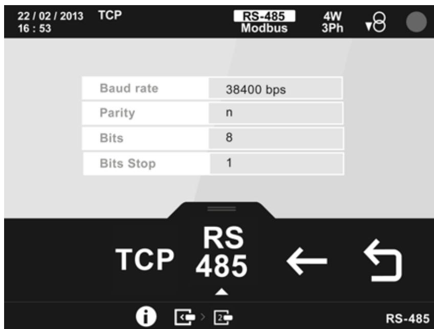
Figura 104: Pantalla de información del módulo Modbus TCP (Bridge) (Pasarela RS-485).
