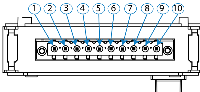
Figura 159: Bornes Entradas/Salidas digitales de Transistor, cara superior.
