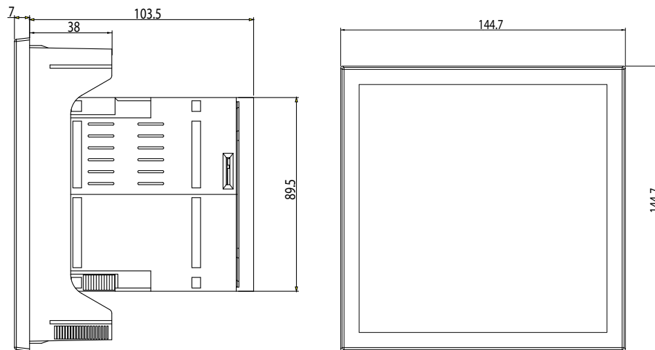
Figura 224: Dimensiones CVM-B150.
