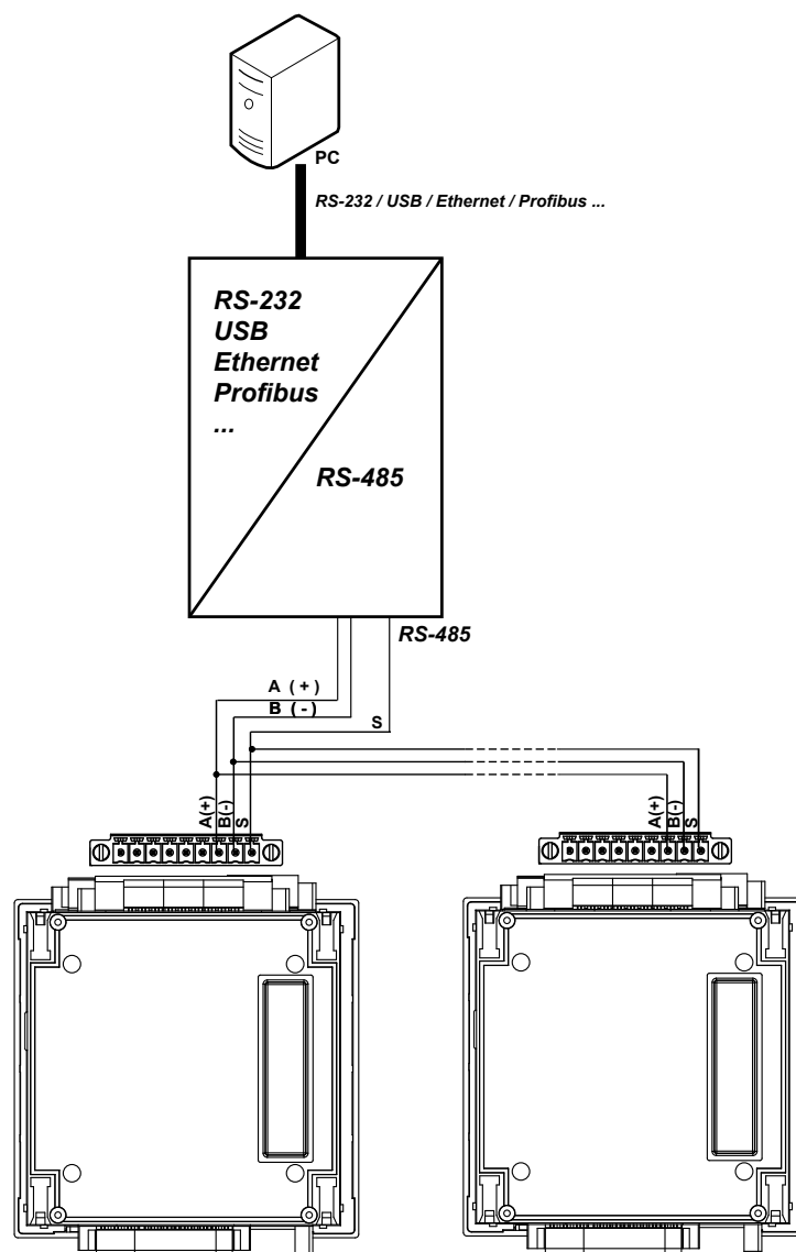
Figura 142: Esquema de conexionado RS-485.
