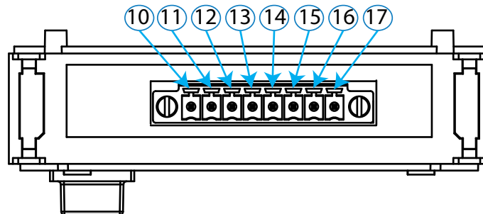
Figura 168:Bornes Entradas/Salidas analógicas, cara inferior.
