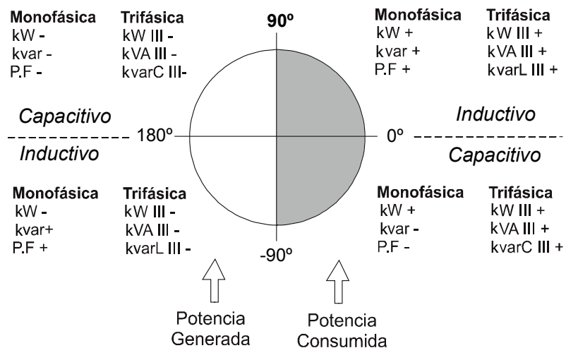
Figura 18: Cuatro cuadrantes de CVM-B.
