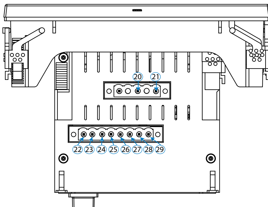
Figura 2: Bornes del CVM-B, cara inferior.
