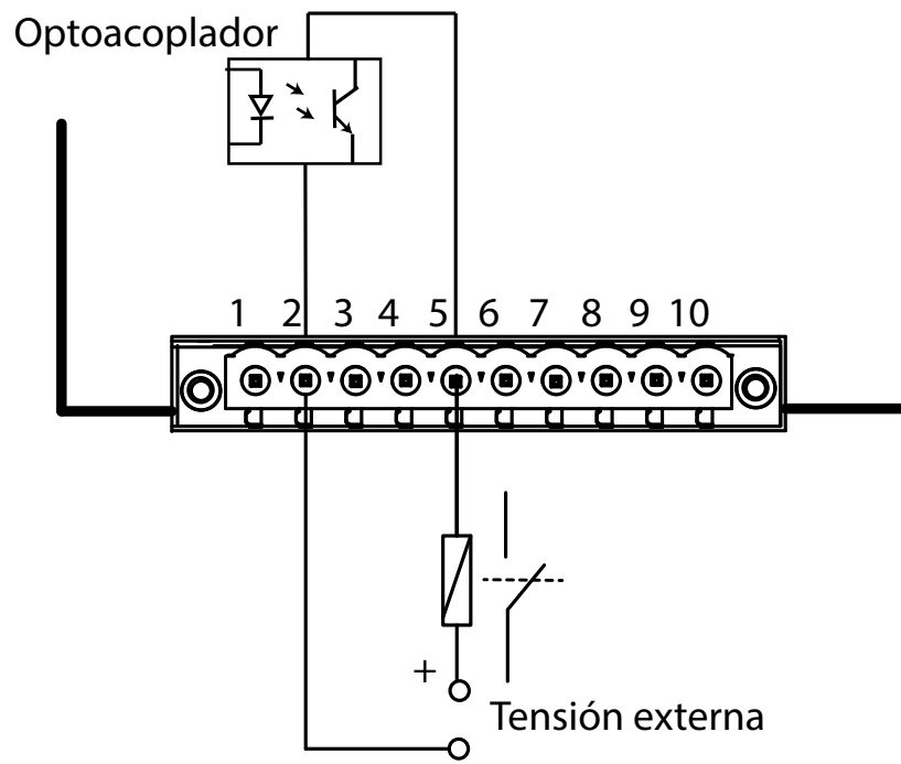
Figura 161: Esquema de conexionado, salida digitales de transistor.
