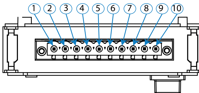
Figura 150: Bornes Entradas/Salidas digitales de Relé, cara superior.
