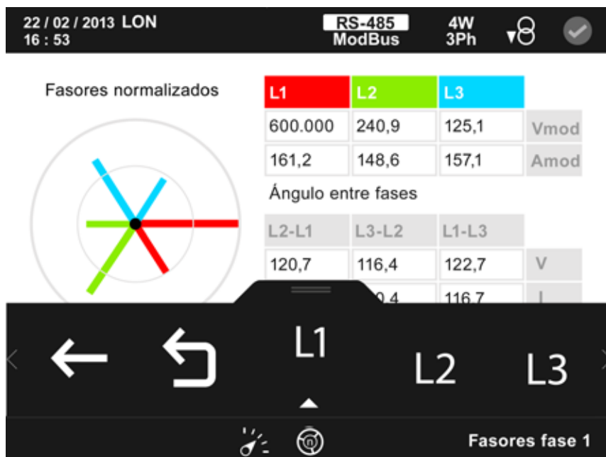
Figura 81: Pantalla de visualización de fasores normalizados.
