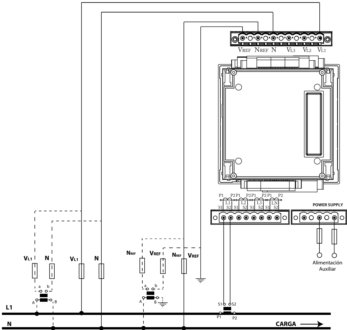
Figura 10: Medida monofásica de fase a neutro de 2 hilos (Secundario del transformador: /1A, /5A o MC1 (/0.250)).
