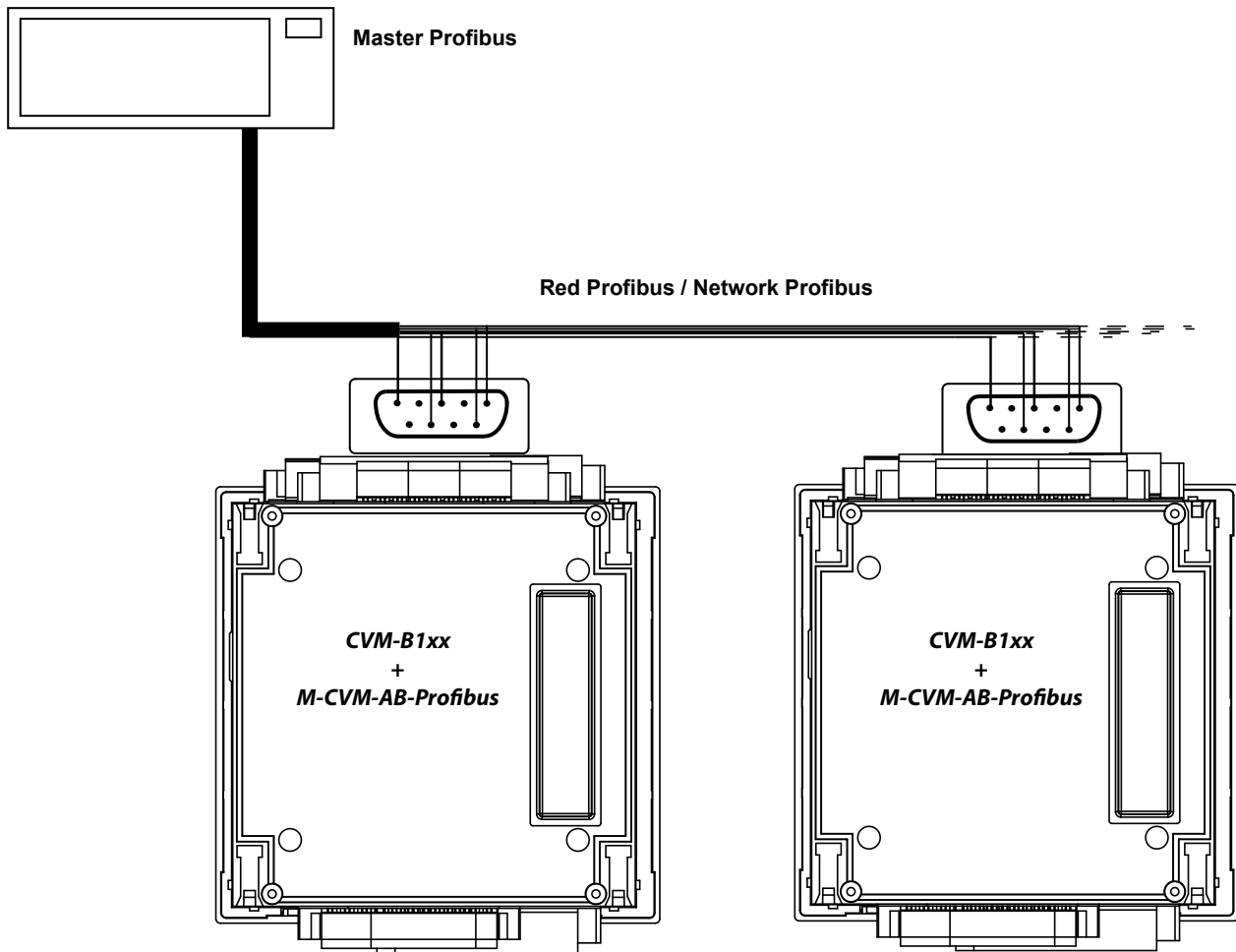
Figura 195:Esquema de conexionado, Profibus.
