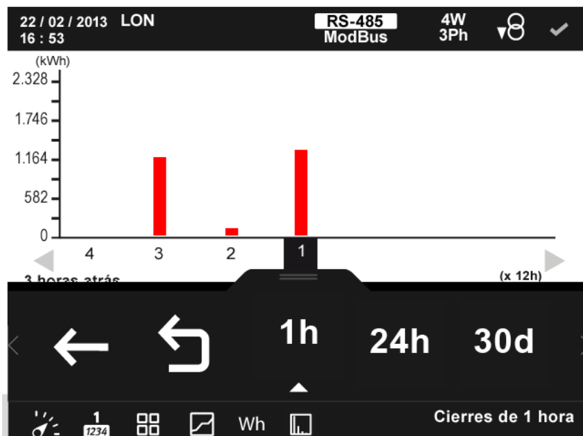
Figura 38: Parámetros incrementales, visualización gráfica ( visualizar 1 parámetro).
