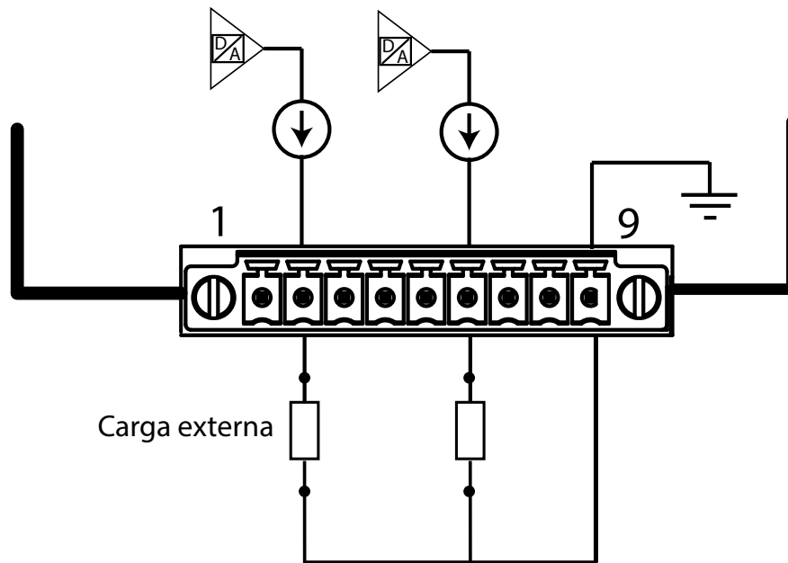
Figura 169: Esquema de conexión, salidas analógicas.
