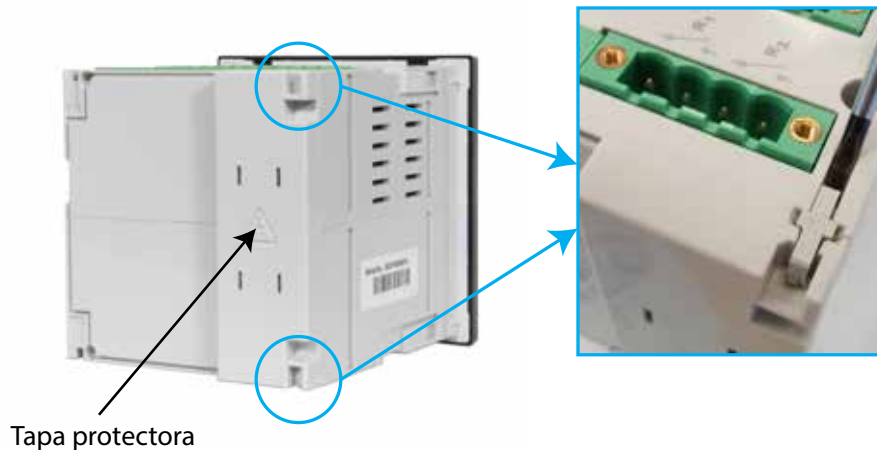
Figura 146: Retirar los 2 clips de sujeción.
