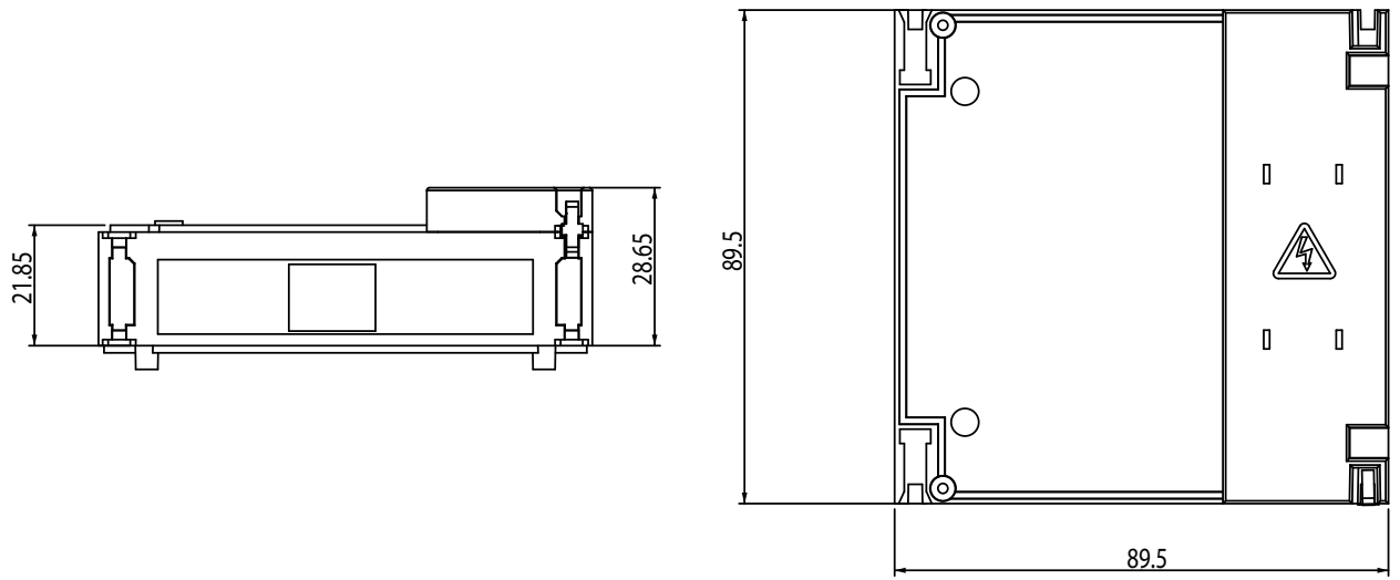
Figura 226: Dimensiones módulo de expansión ( Tapa protectora versión 2).
