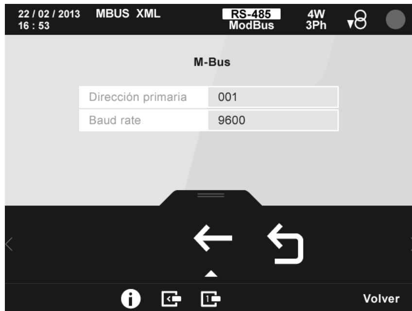
Figura 107: Pantalla de información del módulo MBus.
