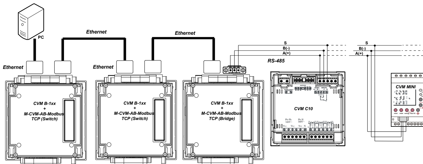
Figura 215: Esquema de conexionado, Modbus TCP (Switch).
