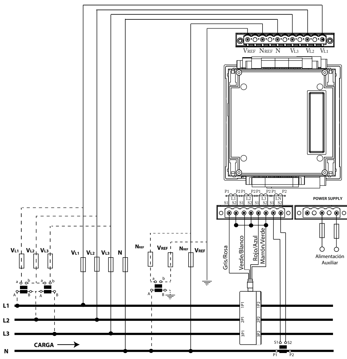
Figura 4: Medida trifásica con conexión a 4 hilos (Transformador tipo MC3 (I0.250)).
