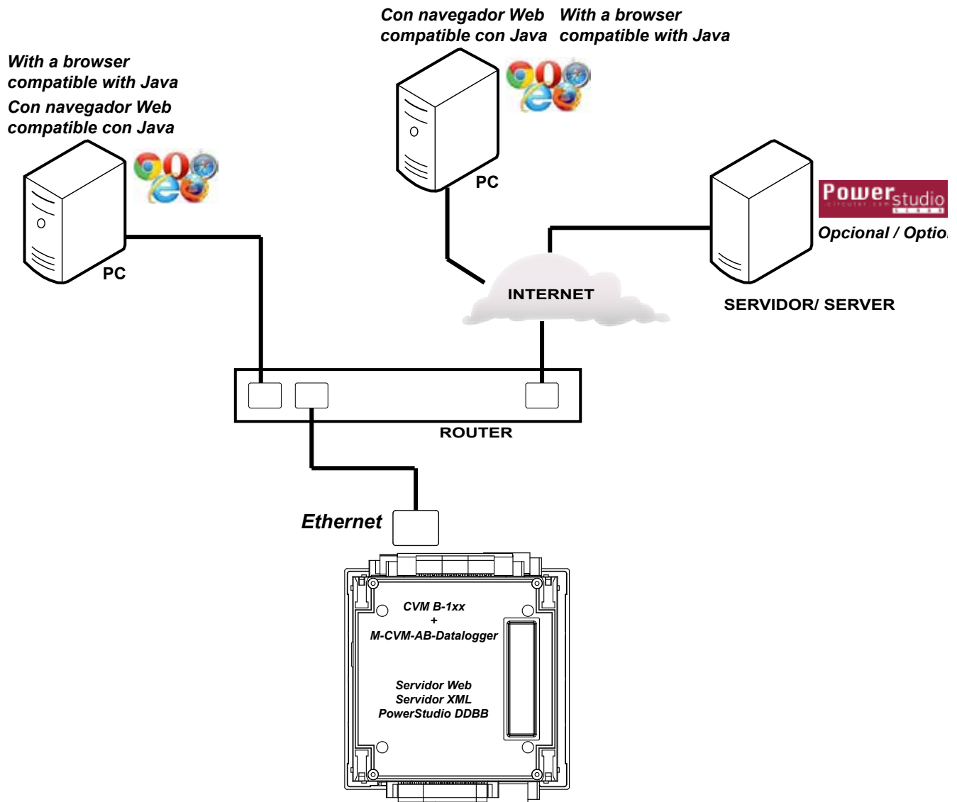
Figura 206:Esquema de conexionado, Modbus Datalogger.
