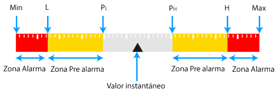
Figura 23: Calculo de la barra gráfica.
