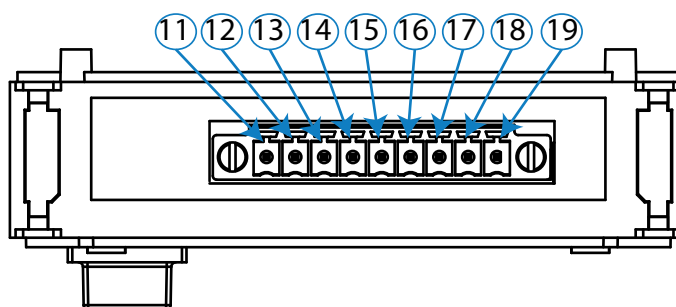
Figura 151: Bornes Entradas/Salidas digitales de Relé, cara inferior.
