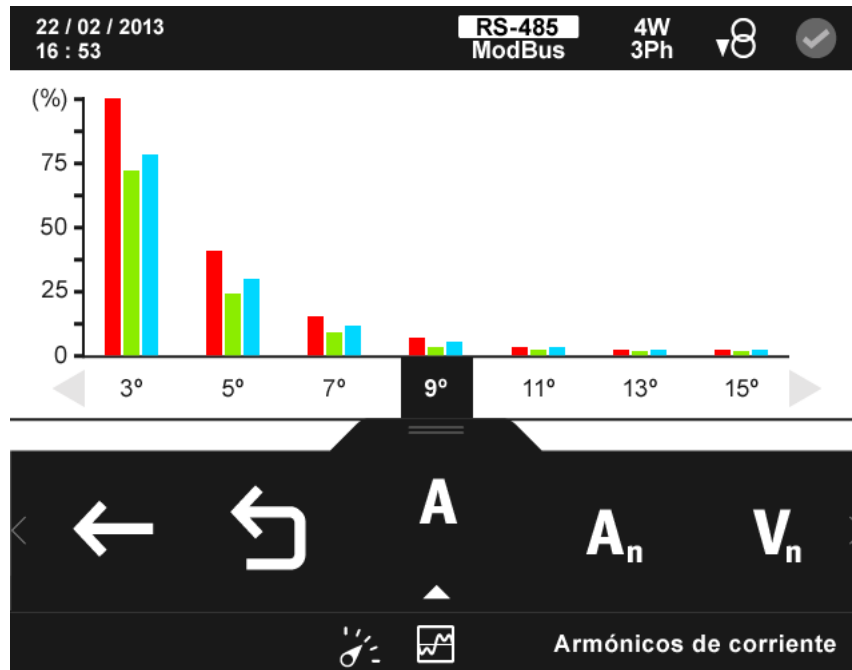
Figura 82: Pantalla de armónicos.
