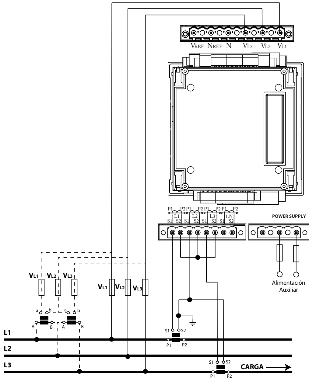
Figura 7: Medida trifásica con conexión a 3 hilos y transformadores en conexión ARON (Secundario del transformador: /1A, /5A o MC1 (/0.250)).
