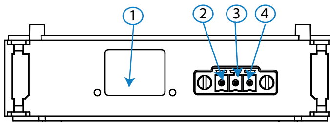
Figura 178: Bornes Módulo de comunicaciones Modbus TCP (Bridge)
