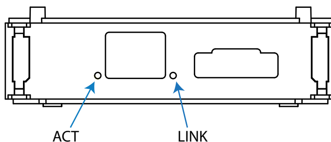
Figura 205: LEDs Modbus Datalogger.
