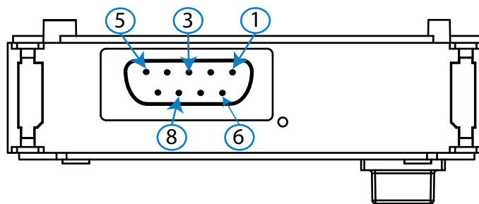
Figura 193: Bornes Módulo de comunicaciones Profibus.
