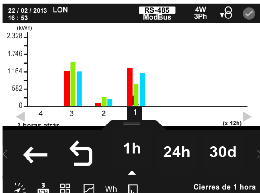
Figura 58: Parámetros incrementales, visualización gráfica (visualizar 3 parámetros).
