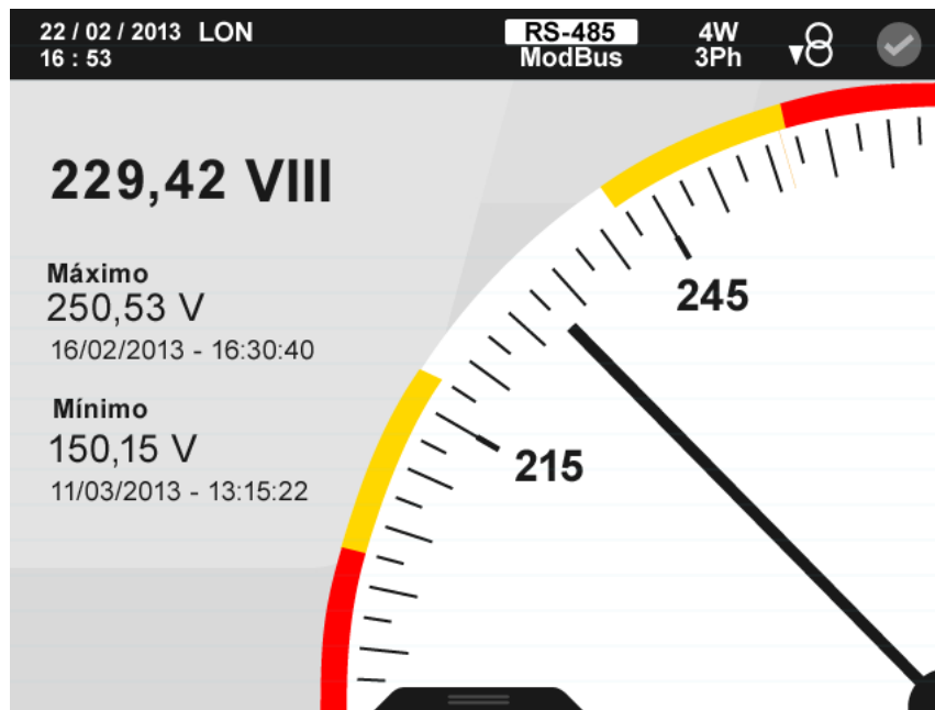
Figura 33: Parámetros instantáneos, visualización analógica ( visualizar 1 parámetro).
