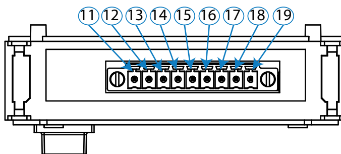
Figura 160:Bornes Entradas/Salidas digitales de Transistor, cara inferior.
