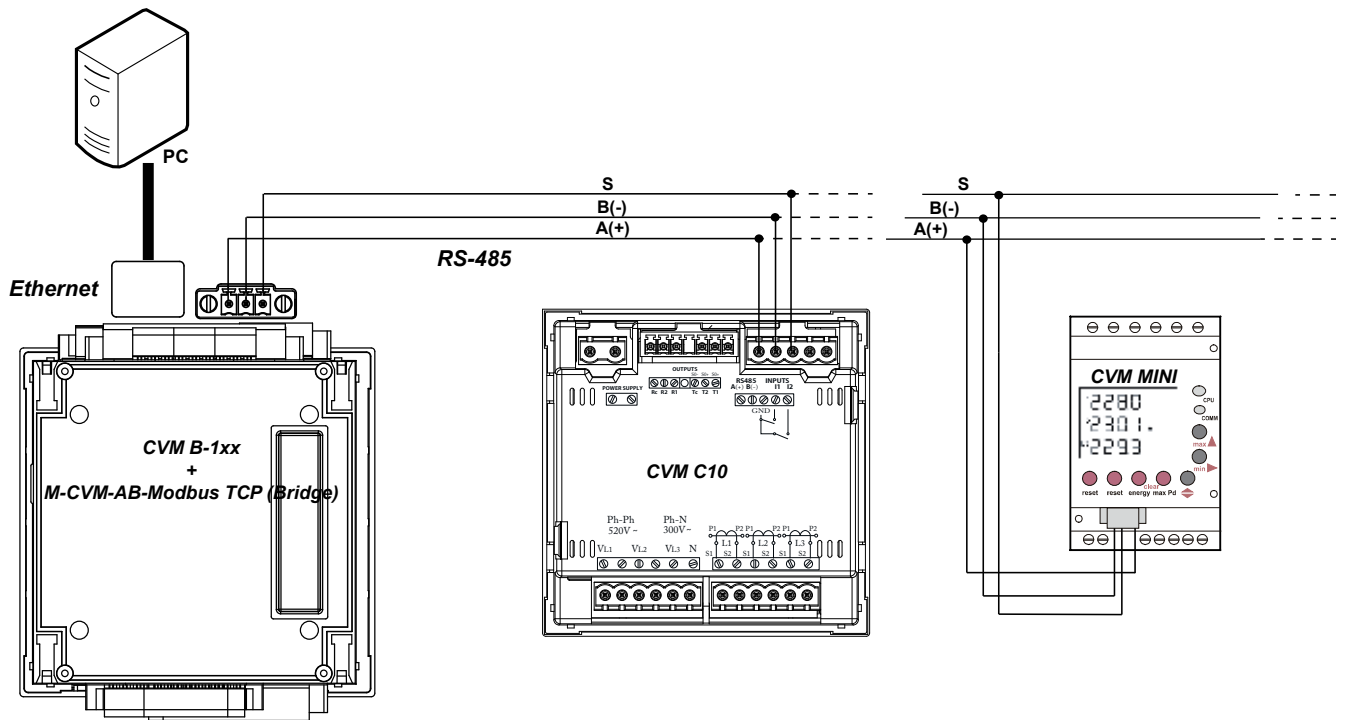
Figura 180:Esquema de conexionado, Modbus TCP (Bridge).
