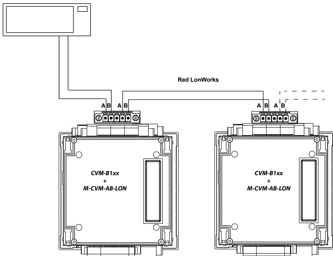
Figura 188:Esquema de conexionado, LonWorks.
