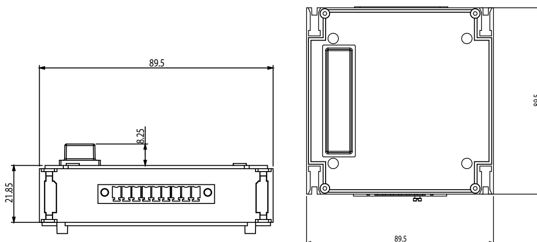
Figura 225: Dimensiones módulo de expansión ( Tapa protectora versión 1).
