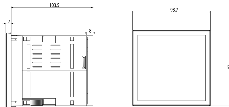
Figura 223: Dimensiones CVM-B100.
