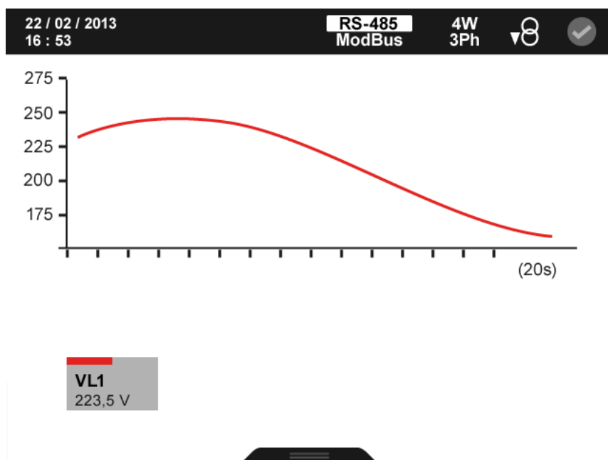
Figura 32: Parámetros instantáneos, visualización gráfica ( visualizar 1 parámetro).
