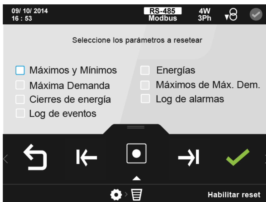
Figura 140: Pantalla de reset de parámetros.
